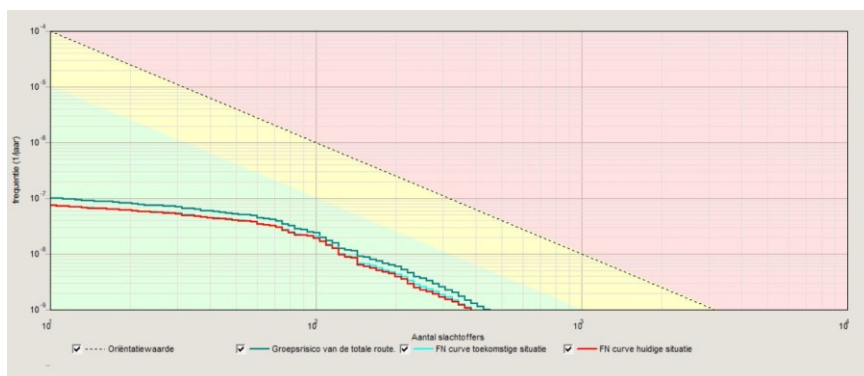
Figuur 7: fN curve spoorlijn Sauwerd – Delfzijl
