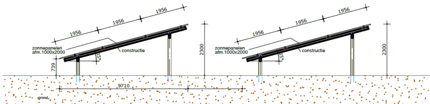
Doorsnede frame/panelen
