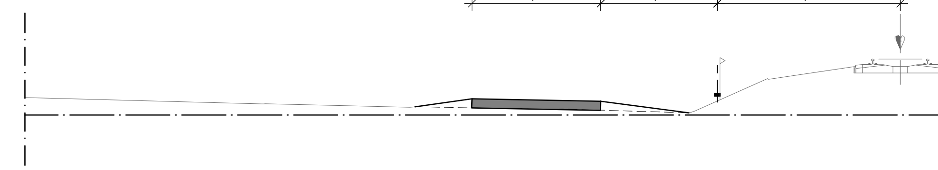
DWARSPROFIEL 2 SCHAAL 1:100
