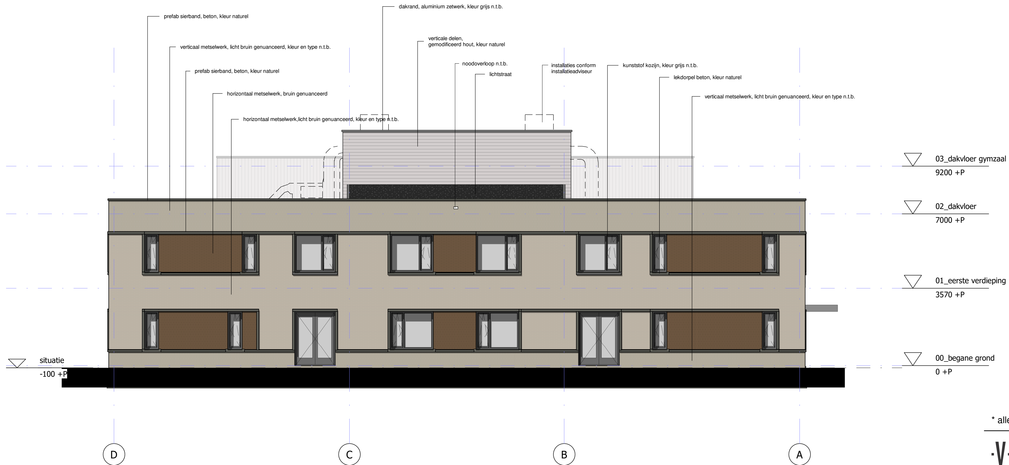
L(--)-202 Linker zijgevel bouwkundig
