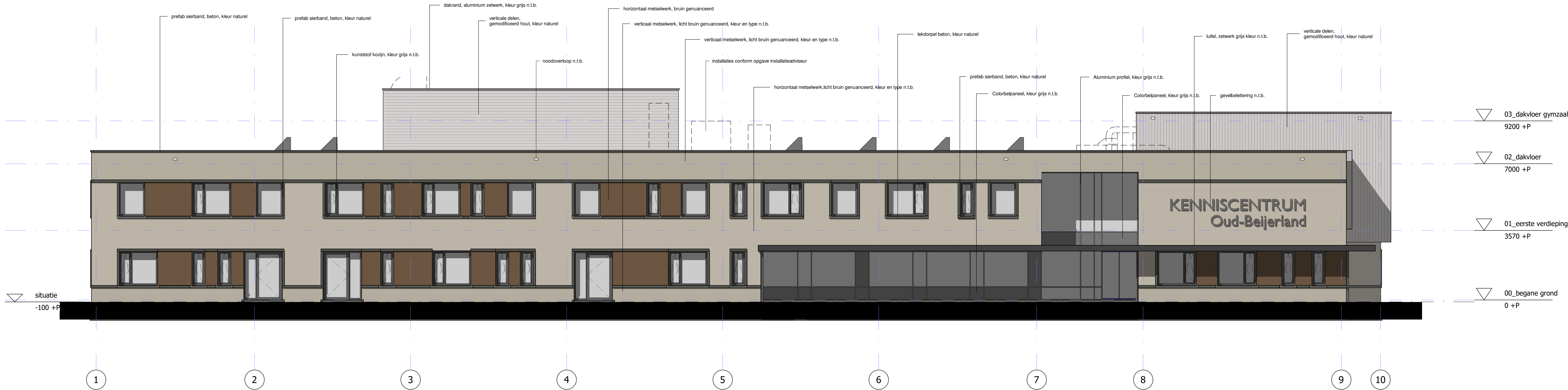
L(--)-201 Voorgevel bouwkundig
