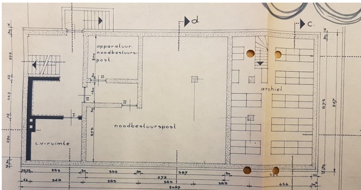
Figuur 16 Plattegrond atoomkelder met o.a. noodbestuurspost en archief (via andere trap bereikbaar)
