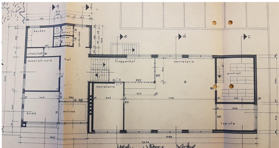
Figuur 5 Plattegrond begane grond met o.a. secretarie en archief
