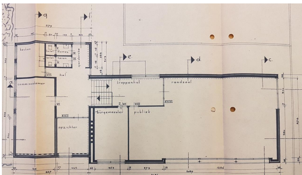
Figuur 6 Plattegrond verdieping met o.a. raadzaal en burgemeesterskamer
