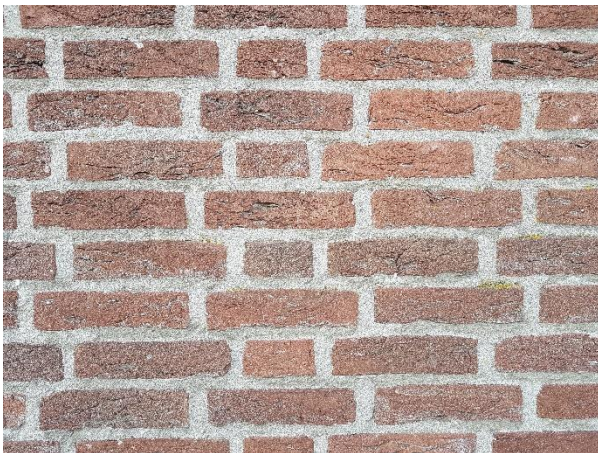
Figuur 8 Detail Schlesischer verband.
