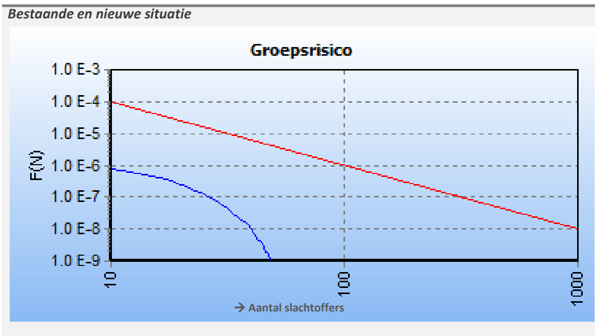
Figuur 6.3 FN curve voor buisleiding W-507-01 van Gasunie voor de kilometer tussen stationing 3400.00 en 4400.00 (bestaande situatie en nieuwe situatie)
