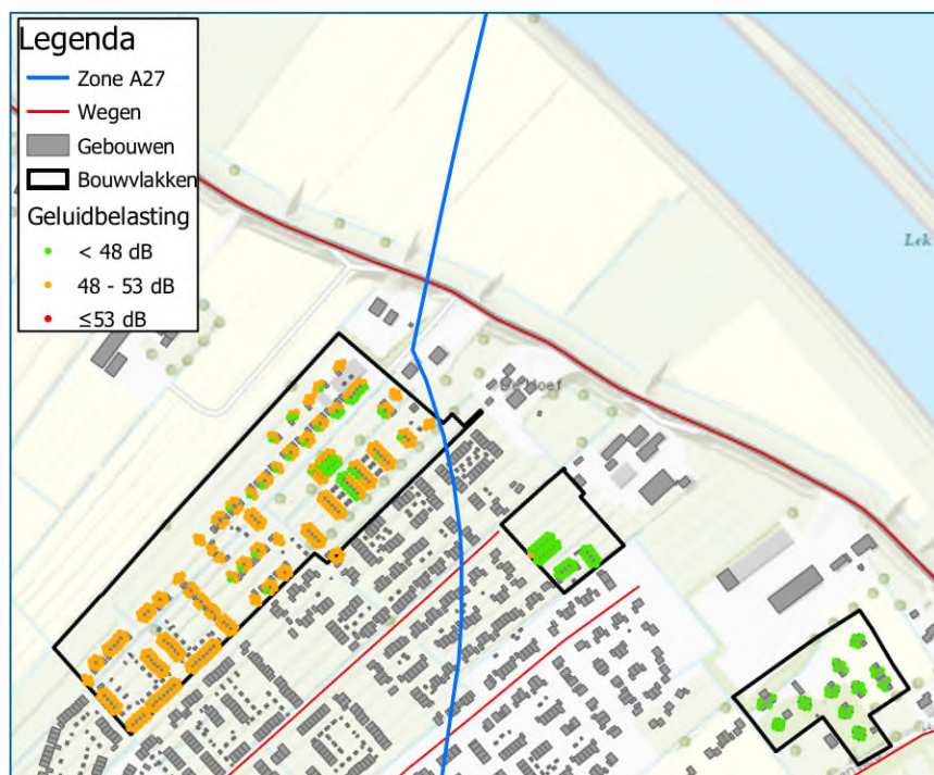
Afbeelding 5.3 Geluidbelasting A27 op 7,5 meter hoogte (incl. aftrek ex art. 110g Wgh)
