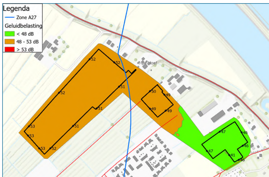
Afbeelding 4.3 Geluidcontour A27 op 7,5 meter hoogte (incl. aftrek ex art. 110g Wgh)
