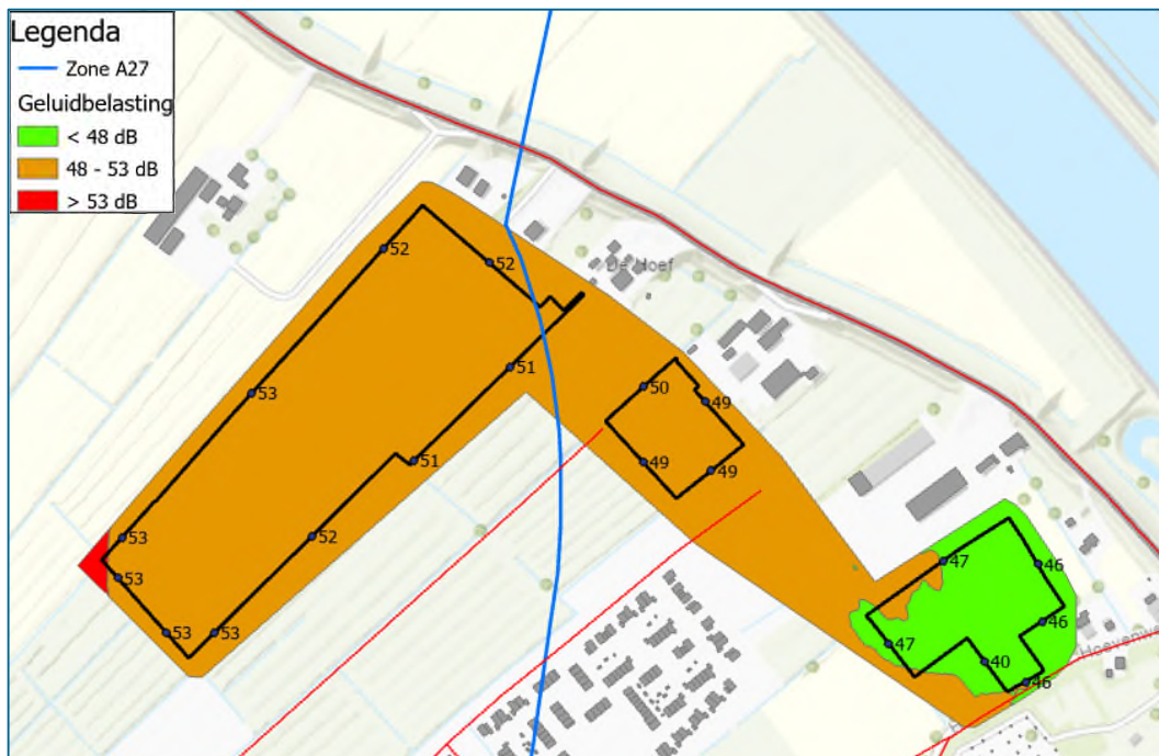
Afbeelding 4.4 Geluidcontour A27 op 10,5 meter hoogte (incl. aftrek ex art. 110g Wgh)
