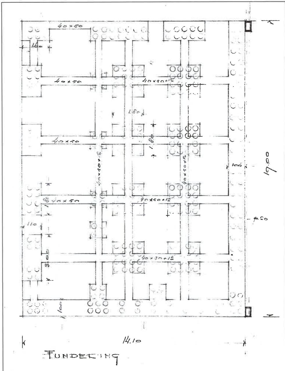
Figuur 5: Bouwtekening van de funderingen van de meelfabriek.
