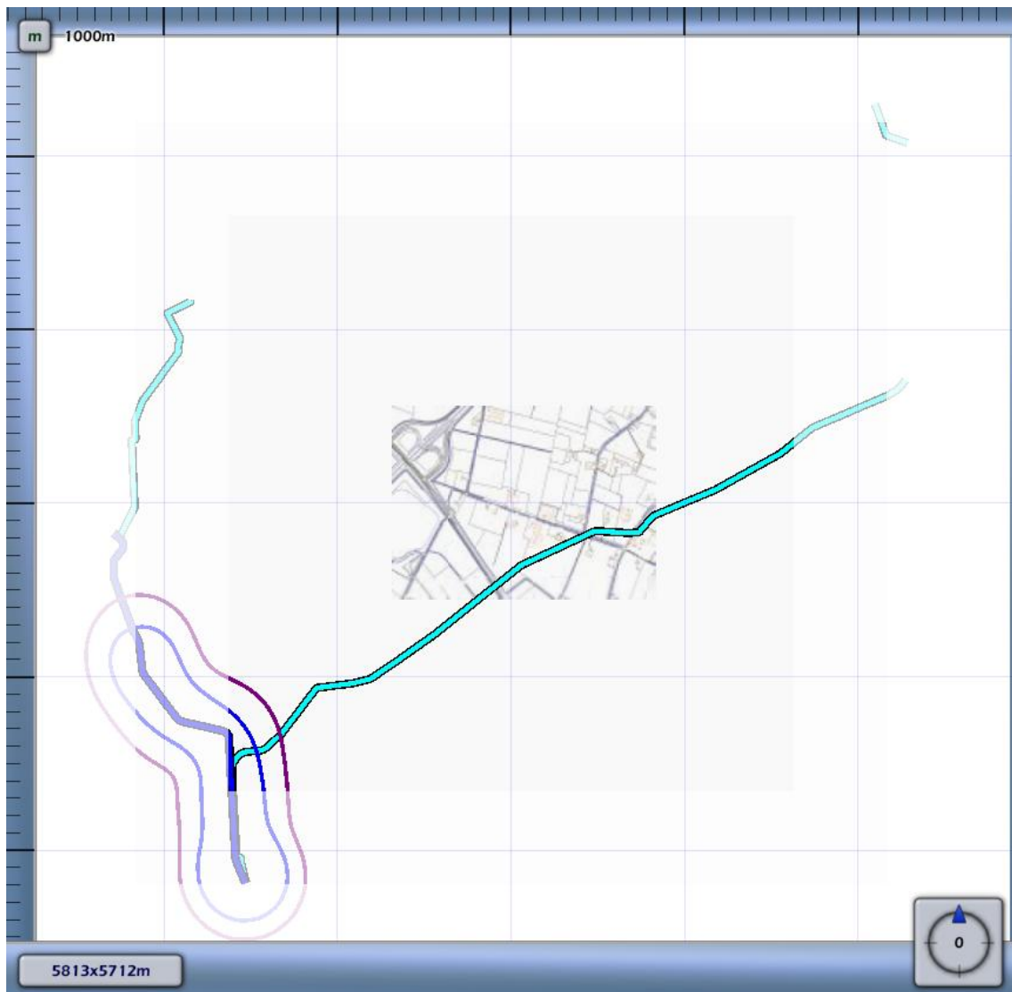
3.1 Figuur 3.1 Plaatsgebonden risico voor A-512 van N.V. Nederlandse Gasunie
