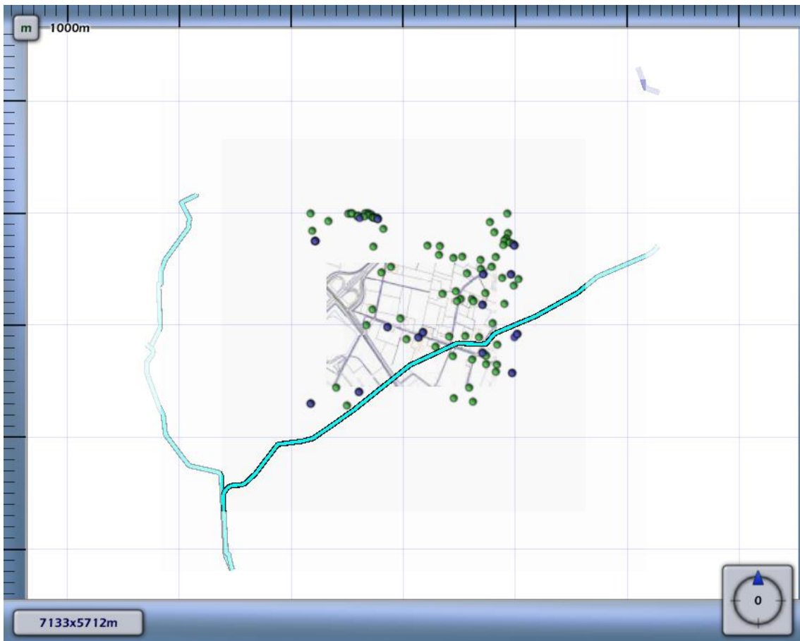
4.4 Figuur 4.4 Groepsrisico screening voor N-566-10 van N.V. Nederlandse Gasunie
