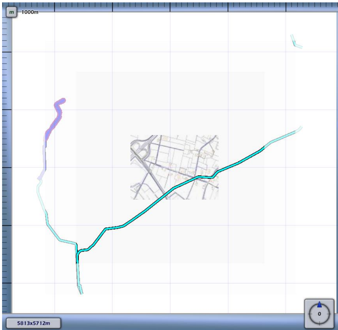
3.4 Figuur 3.4 Plaatsgebonden risico voor N-566-10 van N.V. Nederlandse Gasunie
