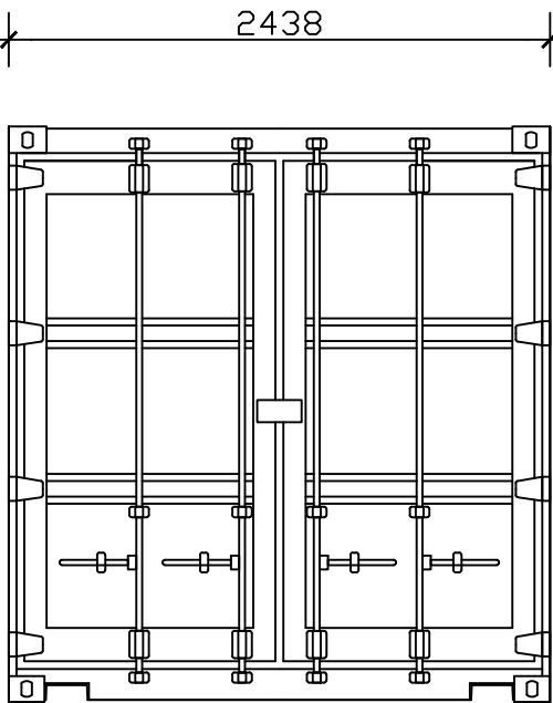
Zijaanzicht vooraan
