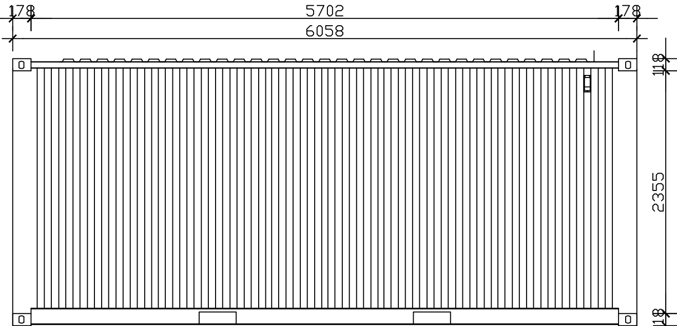
Zijaanzicht links
