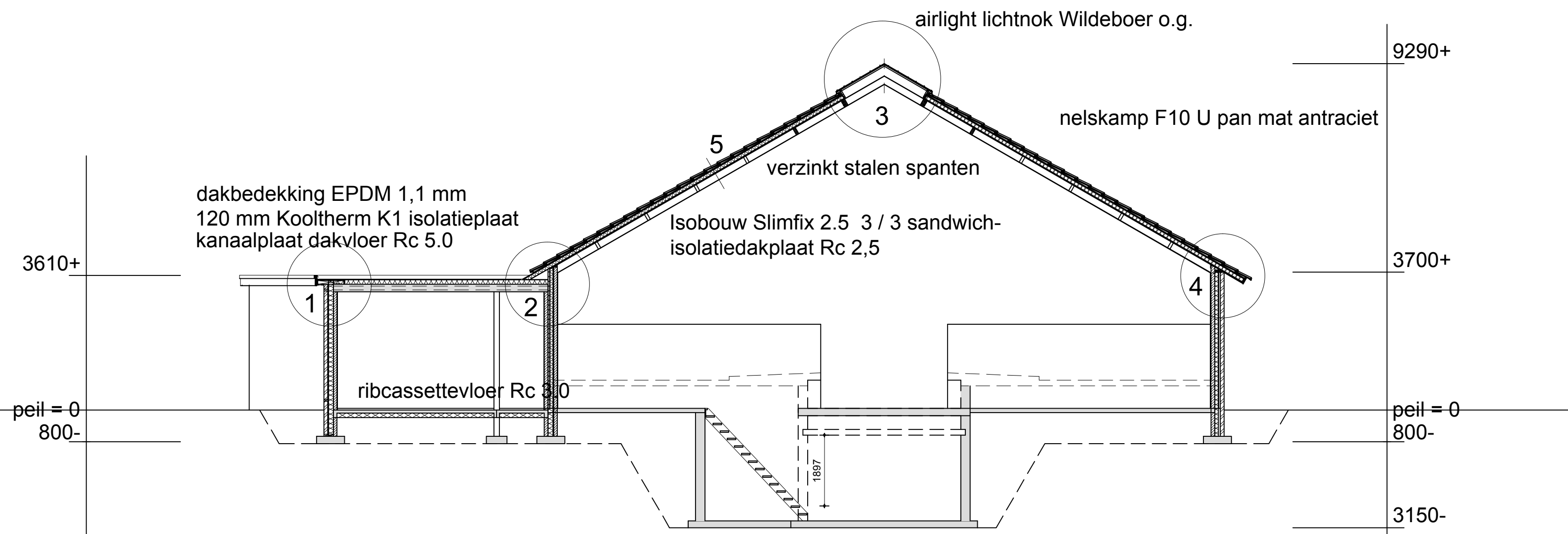
Doorsnede gebouw 6
