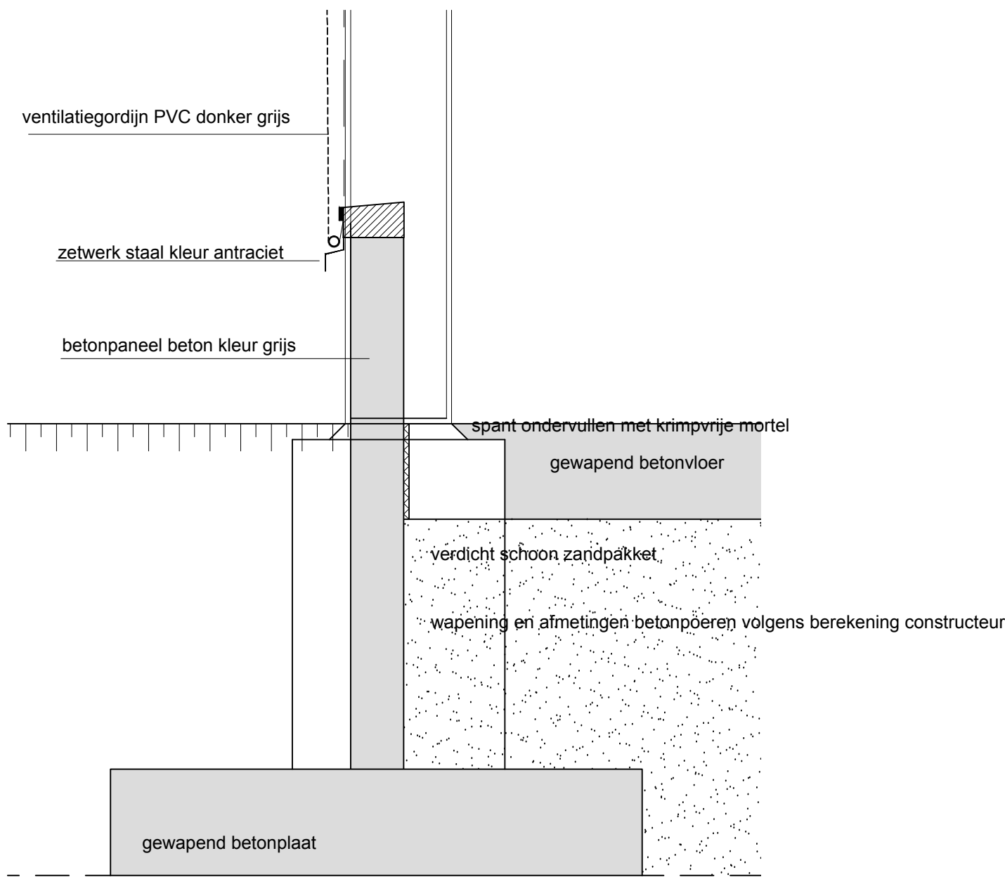
Funderingsdetail 1:10
