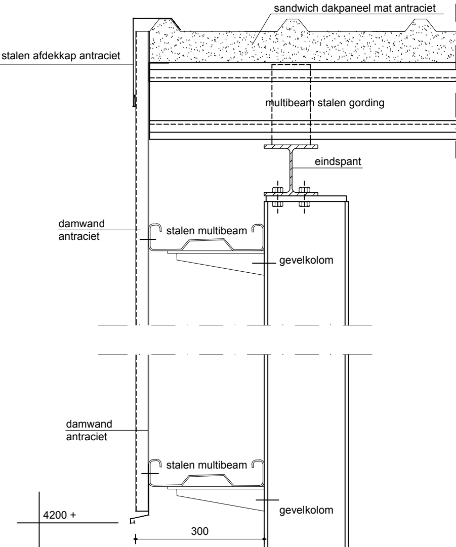
kopgeveldetail 1:10
