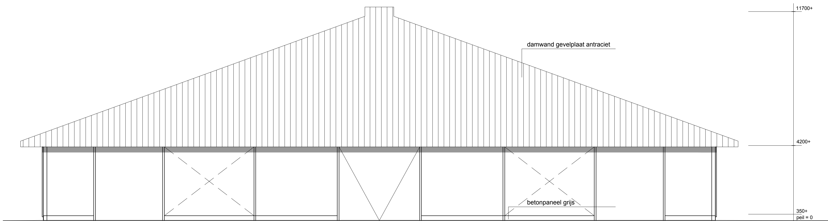
Voor- en achtergevel stal 3 en 4
