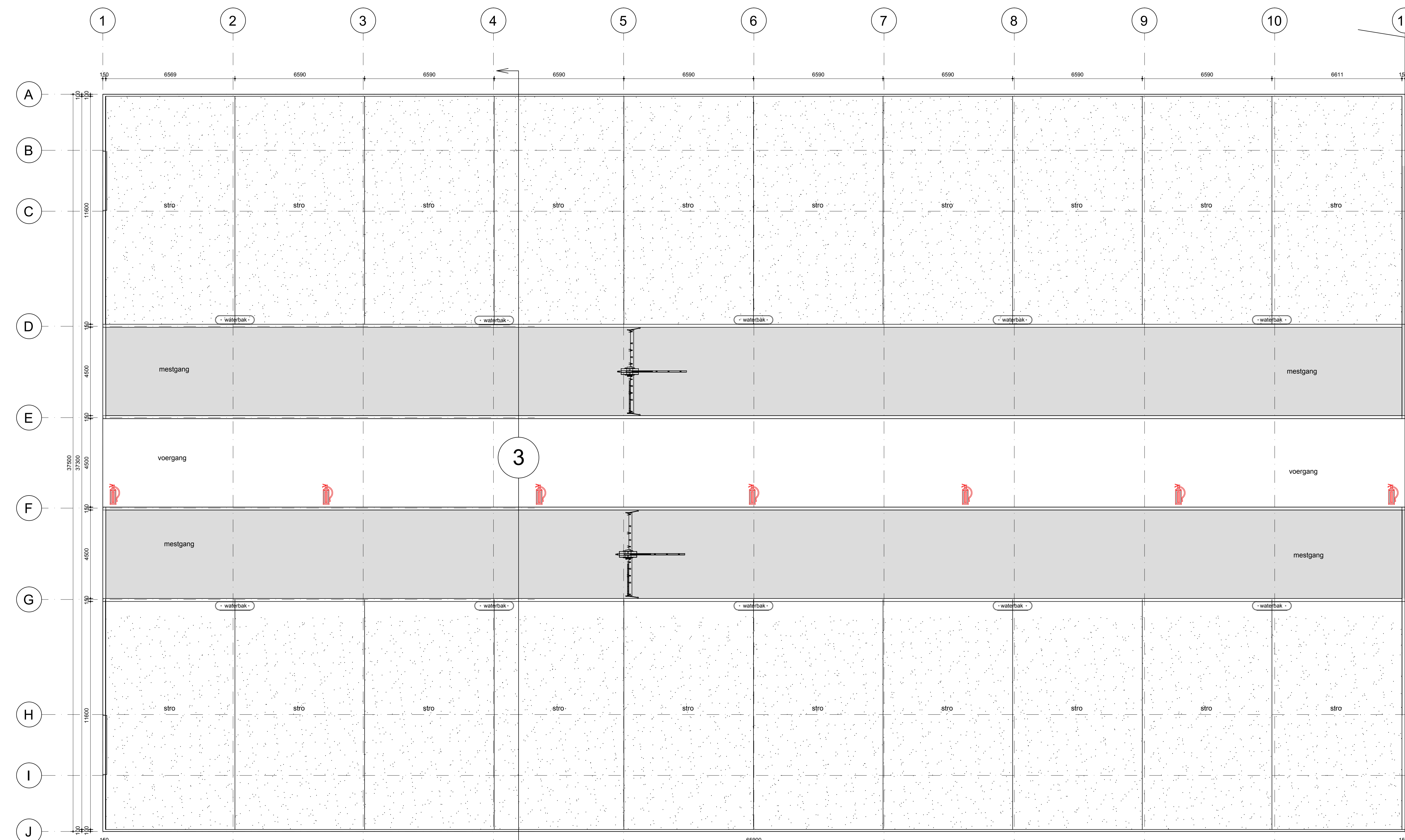
Plattegrond stal 3
