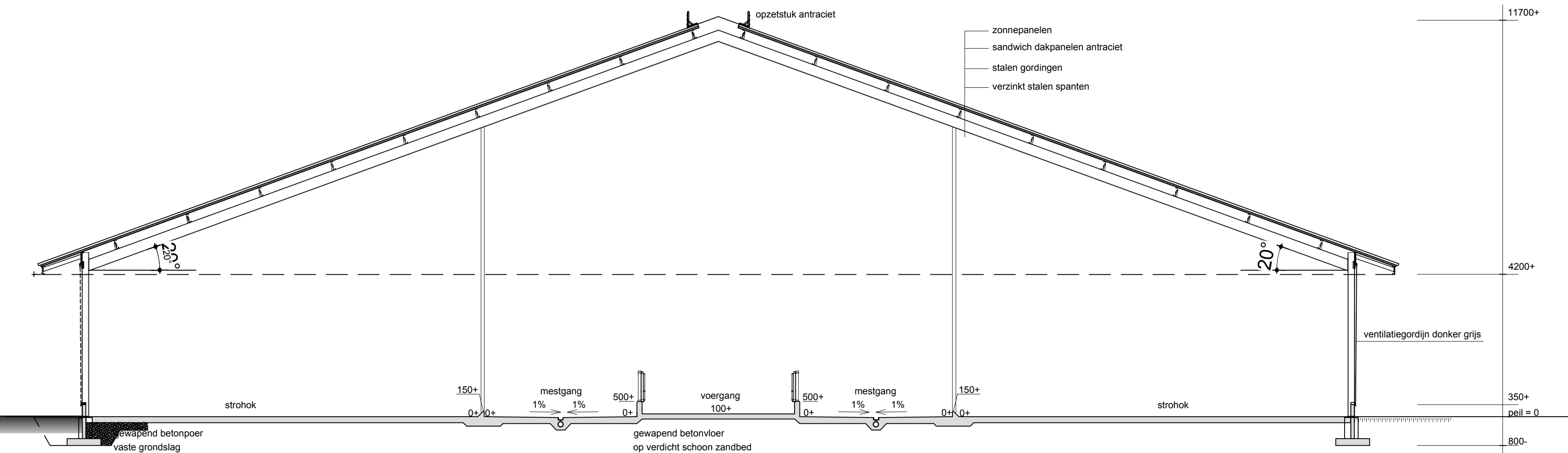
Doorsnede gebouw 3 en 4
