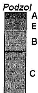
Afbeelding 2. Schematische weergave van een podzolprofiel
