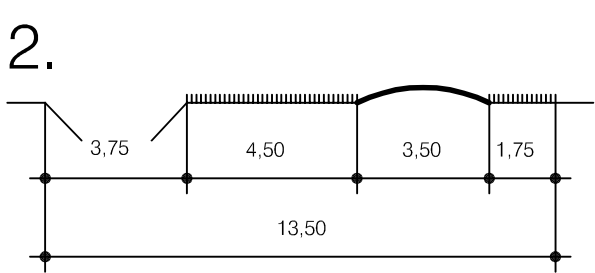
DWARSPROFIEL (schaal 1:200)
