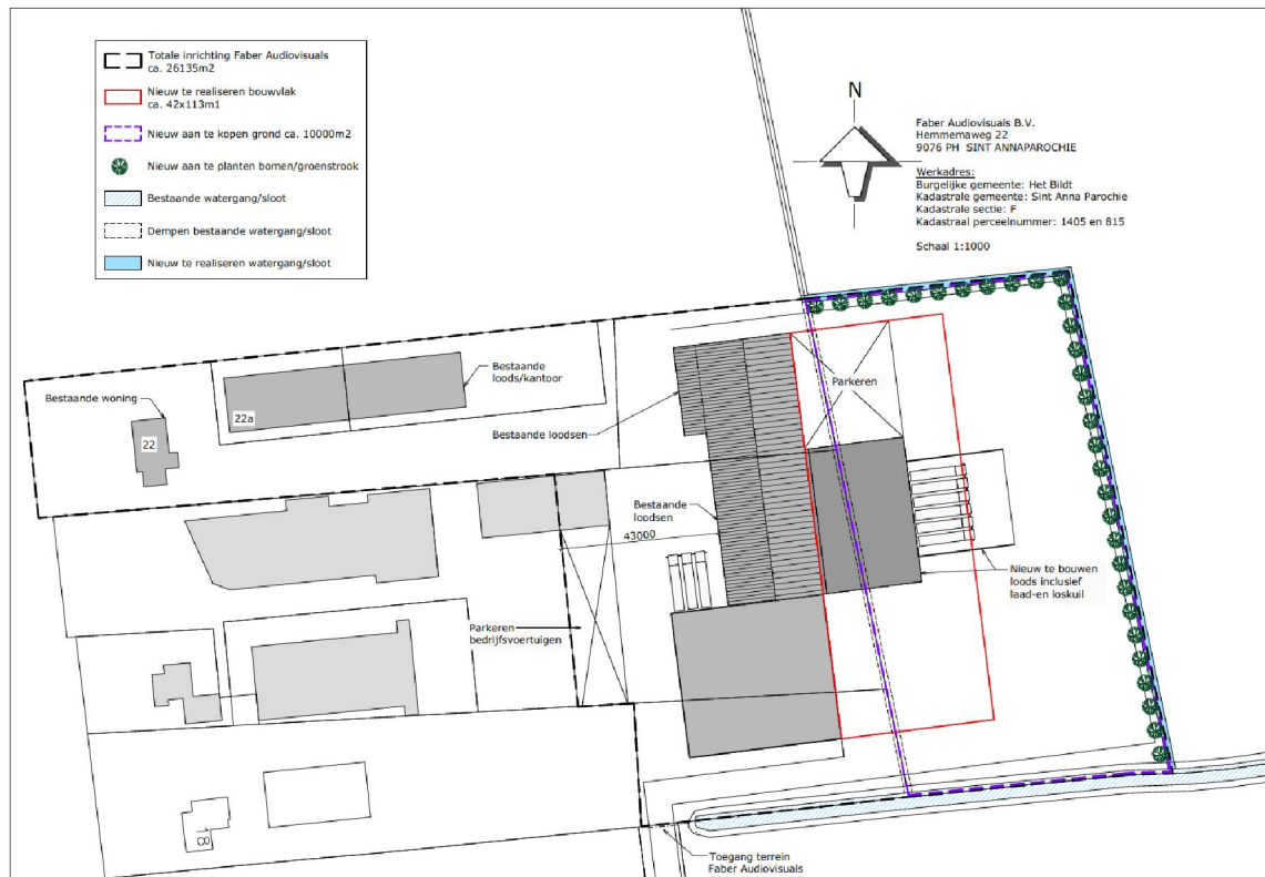
Figuur 3. Impressie van de plannen van de Hemmemaweg 22 te St Annaparochie.
