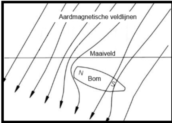
Figuur 14. Principe weergave werking passieve NON realtime oppervlakedetectie/ magnetometrie.
