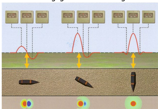
Figuur 16. Visuele weergaven resultaten passieve NON realtime oppervlakedetectie.
