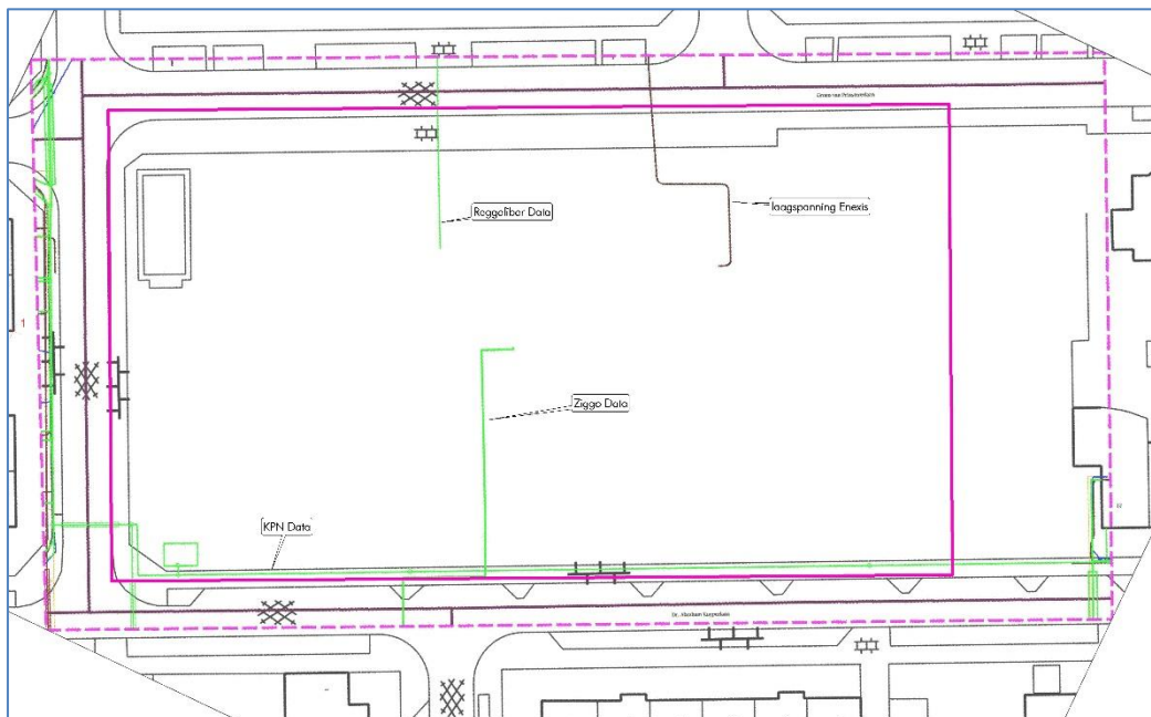
Afbeelding 2 - Weergave van kabels en leidingen ter plaatse van het projectgebied. Roze: begrenzing projectlocatie. Groen: datakabels. Bruin: spanningskabels.
