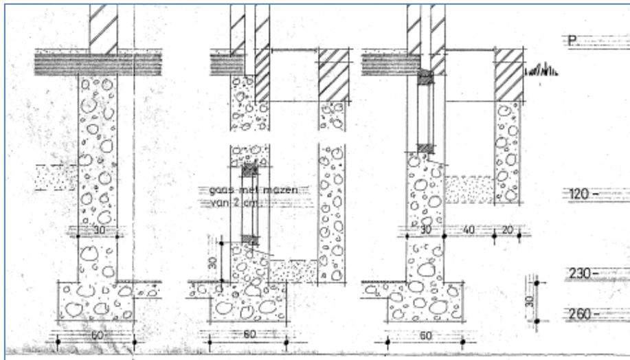
Afbeelding 32 – Voorbeeld fundering kelder voormalige Franciscusschool. Hierop is onder andere te zien tot welke diepte de funderingspalen van de kelder in de grond zitten.
