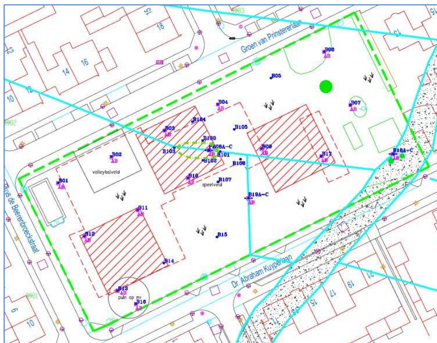
Afbeelding 13 – Uitsnede bodemonderzoek Verhoeven Milieutechniek B.V. Groene stippellijn: Interventiewaardecontour PAK in grond. Rode stippellijn: voormalige bebouwing. Rode arcering: toekomstige bebouwing. Blauw: boringen.
