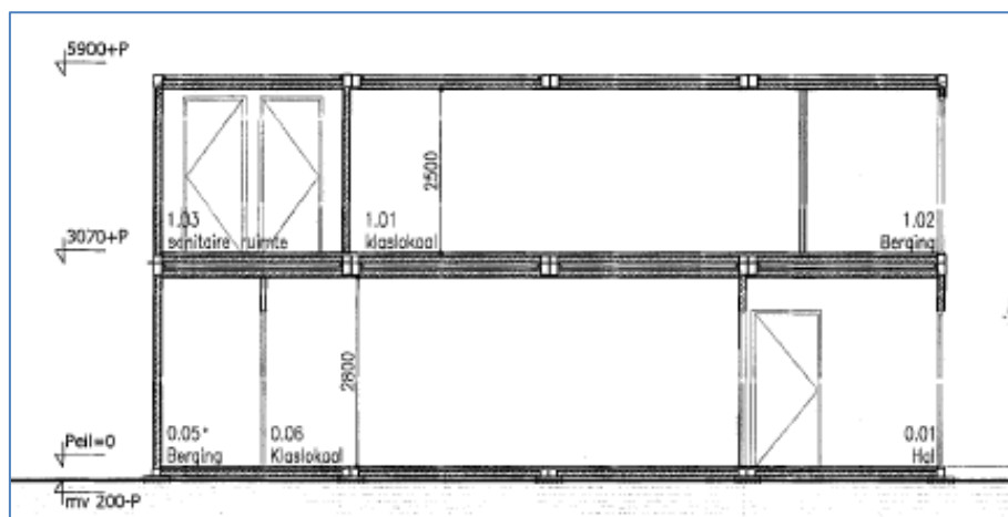
Afbeelding 33 – Units ten westen van de Franciscusschool. Linksonder in de afbeelding is aangegeven tot welke diepte de units in de grond zitten.
