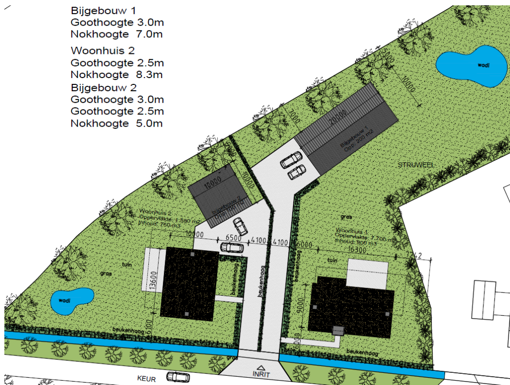
Figuur 4. Onderzoekslocatie met schets bouwplan (bron: Omni architecten)
