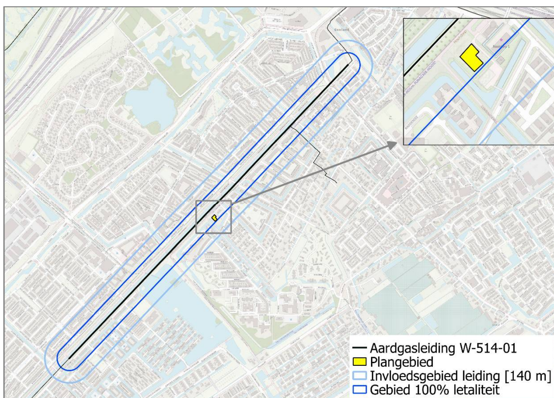
Figuur 2. Aardgasleiding W-514-01 en invloedsgebied
