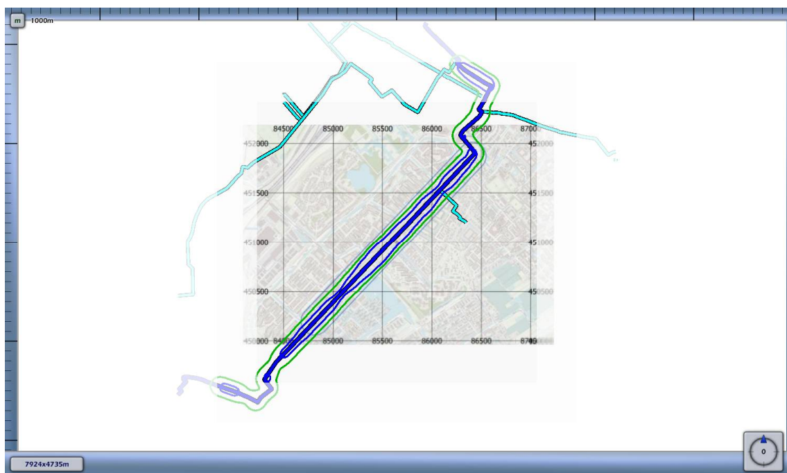
3.1 Figuur 3.3 Plaatsgebonden risico voor 5226_leiding-W-514-01-deel-1 van N.V. Nederlandse Gasunie
