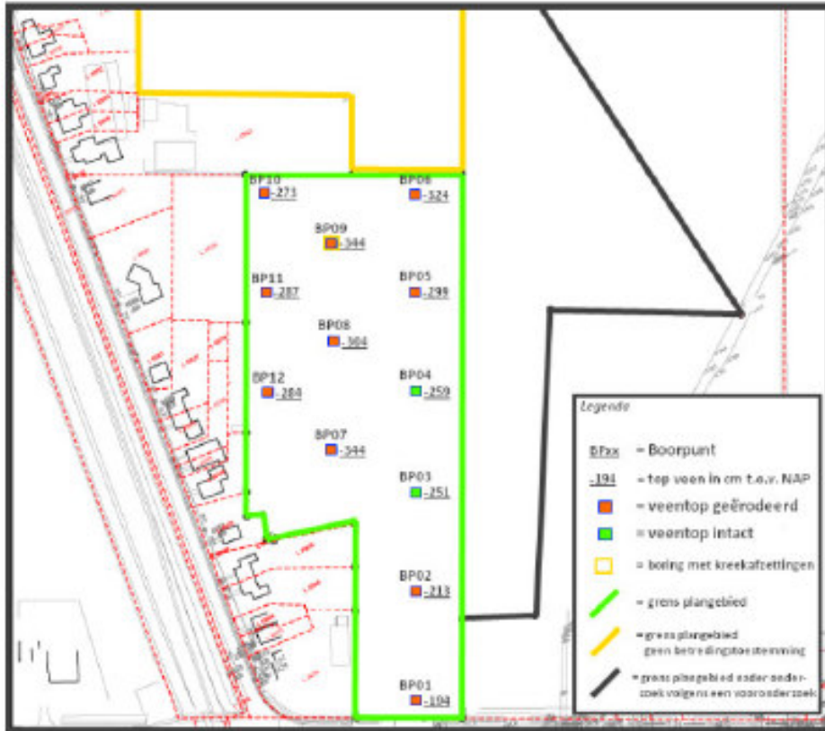
Figuur 2: Booronderzoek Zuidwestelijk perceel
