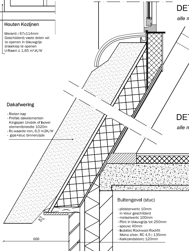
DETAIL V01 / SCHAAL 1:20
