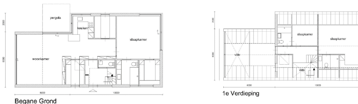
Figuur 5. Plattegrond schuurwoning. (Bron: architect X)
