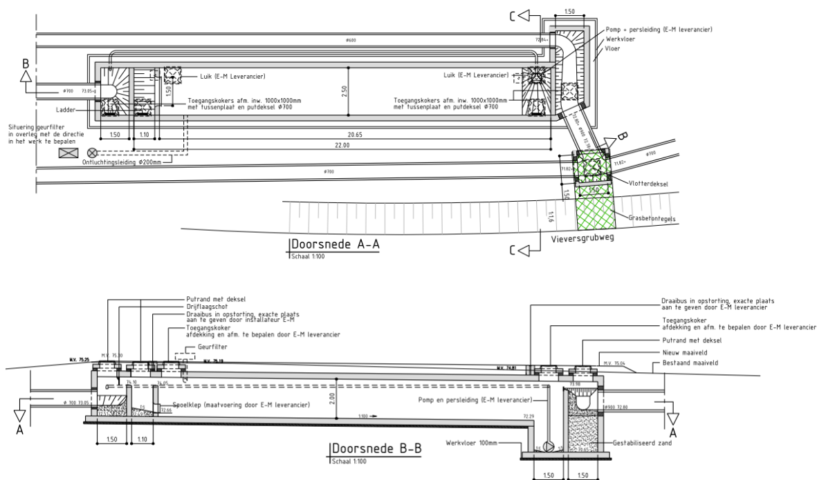
Afbeelding 4: Principe tekening bergbezinkbassin (bovenaanzicht en dwarsdoorsnede)
