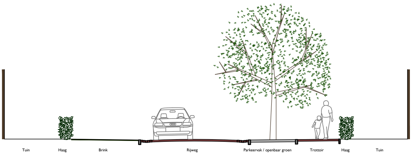
Principeprofiel A-A
