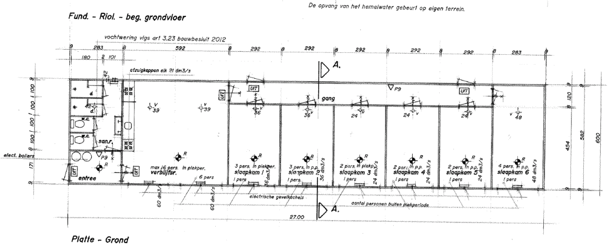
Figuur 6. Bouwtekening huisvesting
