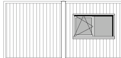
Zijaanzicht (schaal 1:100)
