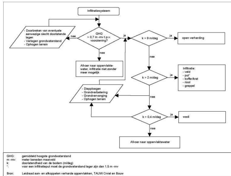
Figuur I. Beslismethodiek infiltratietechniek
