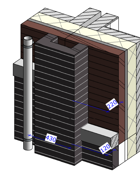
06. detail boekensteun
