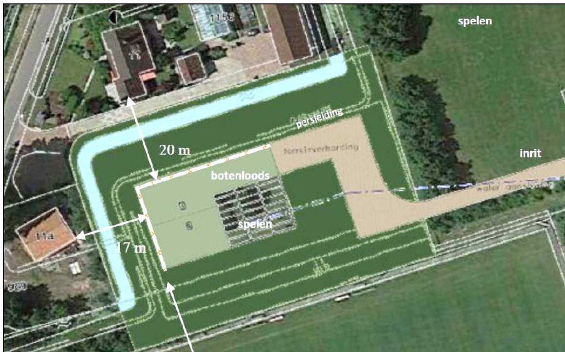
Figuur 3. Plansituatie van het scoutingterrein op sportpark te Den Hoorn.
