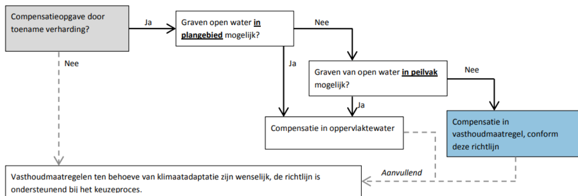
Figuur 5: Stroomschema toepassen van vasthoudmaatregelen (Bron: Richtlijn toepassen vasthoudmaatregelen ter compensatie van verharding in het watertoetsproces, Delfland)
