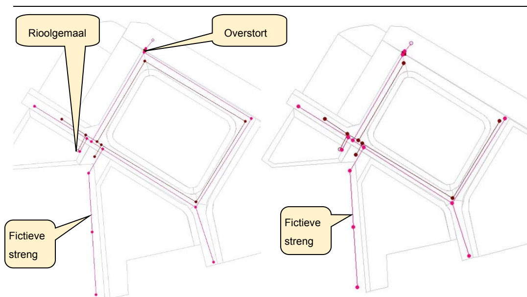
Figuur 4.9 Structuur rioelstelsel variant 1 en 2, beide inclusief uitbreiding
