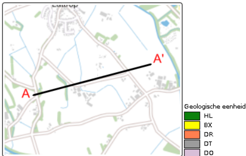
Figuur 1 Geologisch opbouw landelijk model DGM v2.2
