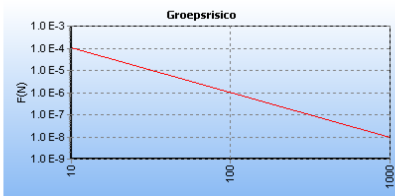
5.5 Figuur 5.5 FN curve voor Z-514-15 van N.V. Nederlandse Gasunie voor de kilometer tussen stationing 0.00 en stationing 0.00
