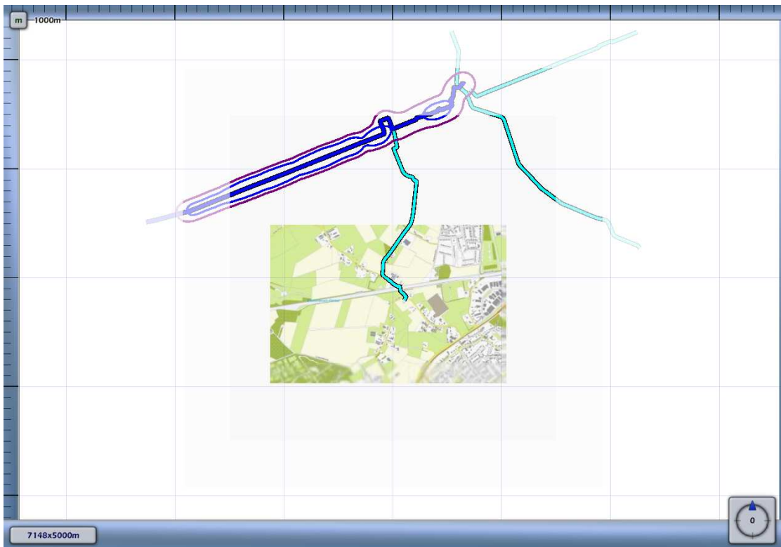
3.5 Figuur 3.5 Plaatsgebonden risico voor Z-514-15 van N.V. Nederlandse Gasunie
