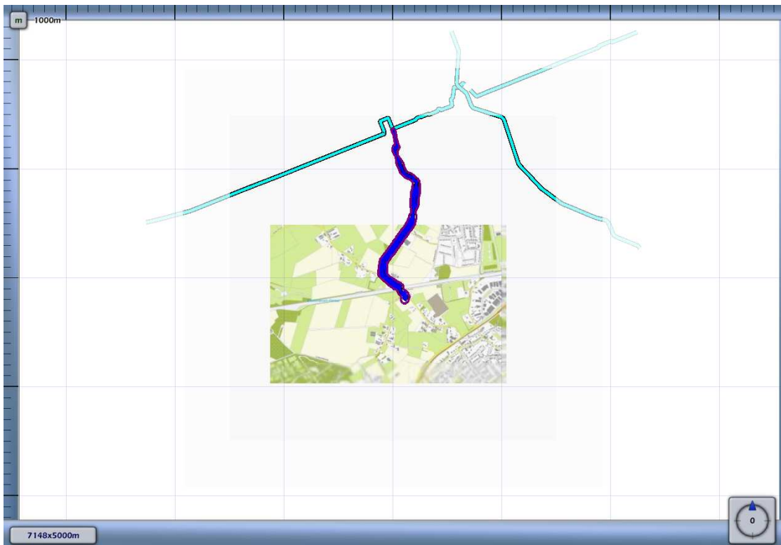
3.3 Figuur 3.3 Plaatsgebonden risico voor Z-514-03 van N.V. Nederlandse Gasunie
