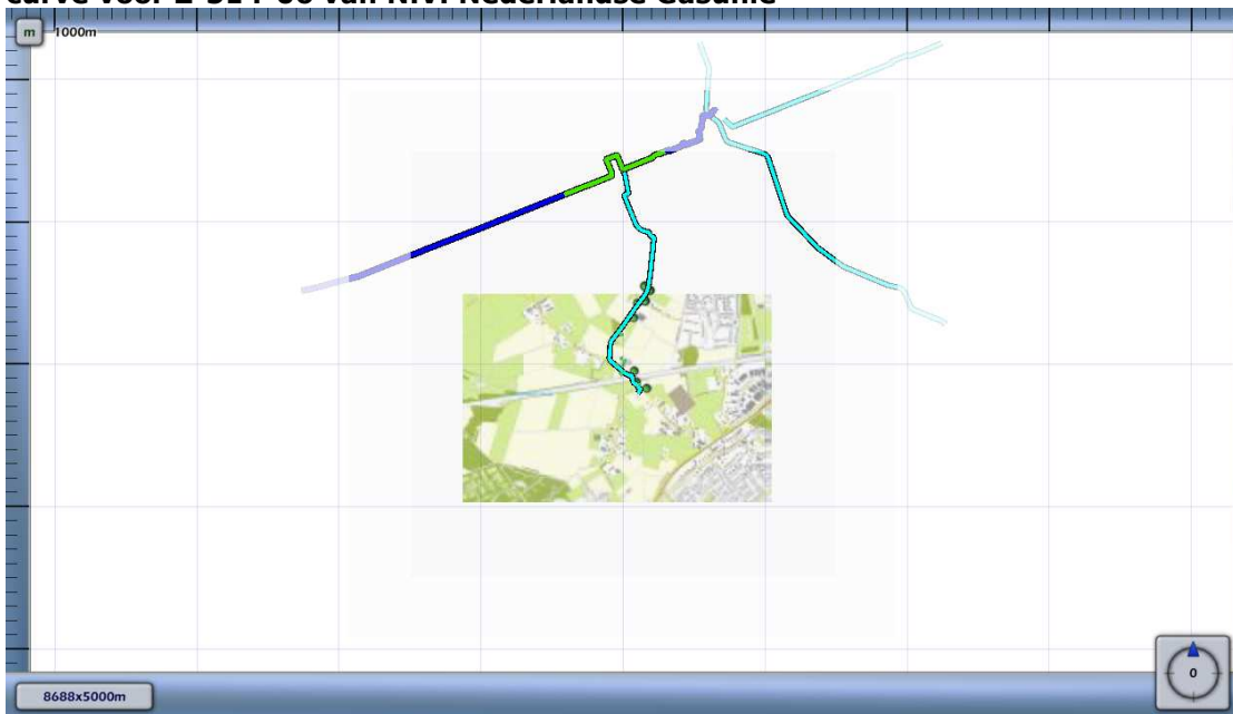
Figuur 4.4 Kilometer leiding behorende bij de maximale overschrijding van de FN-curve voor Z-514-06 van N.V. Nederlandse Gasunie
