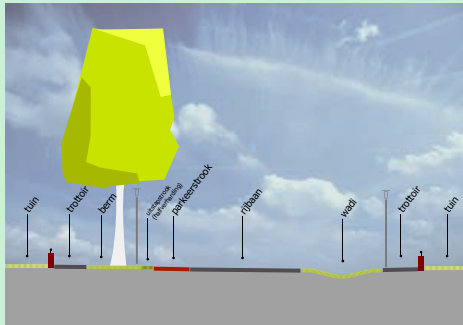
Principeprofiel lanen
