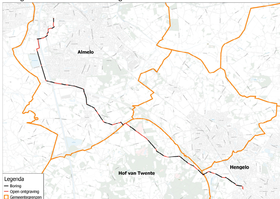
Figuur 1.1: Overzichtskartaal ondergrondse 110kV kabelverbinding Almelo Mosterdpot (AMLM) - Hengelo Weideweg (HGLW)
