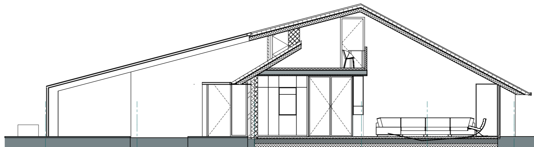
Doorsnede C-C
