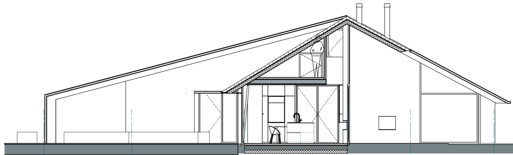
Doorsnede B-B
