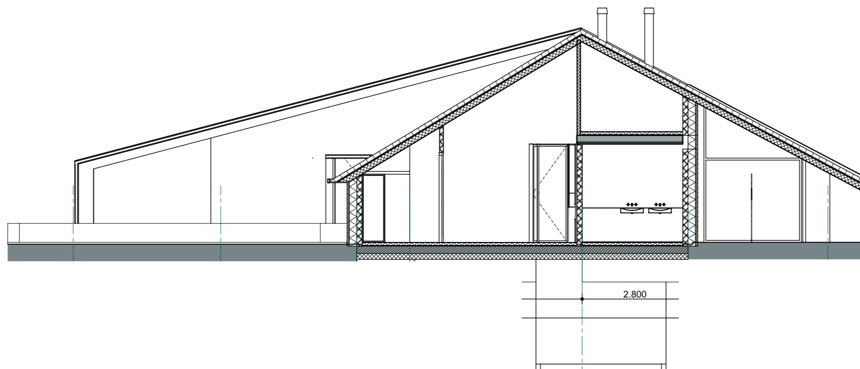
Doorsnede D-D
