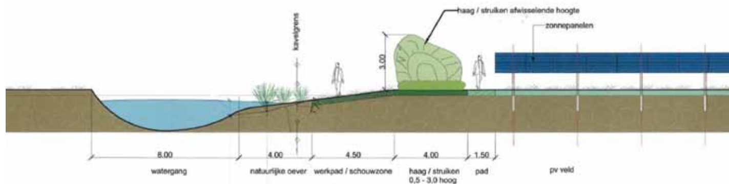
profiel natuurvriendelijke oever na de werkzaamheden
