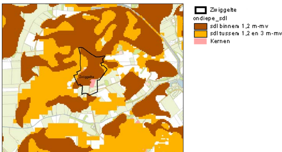
Figuur 9. Slechtdoorlatende lagen
