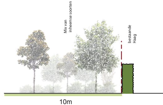
Profiel Hakhoutbosje schaal 1:200
