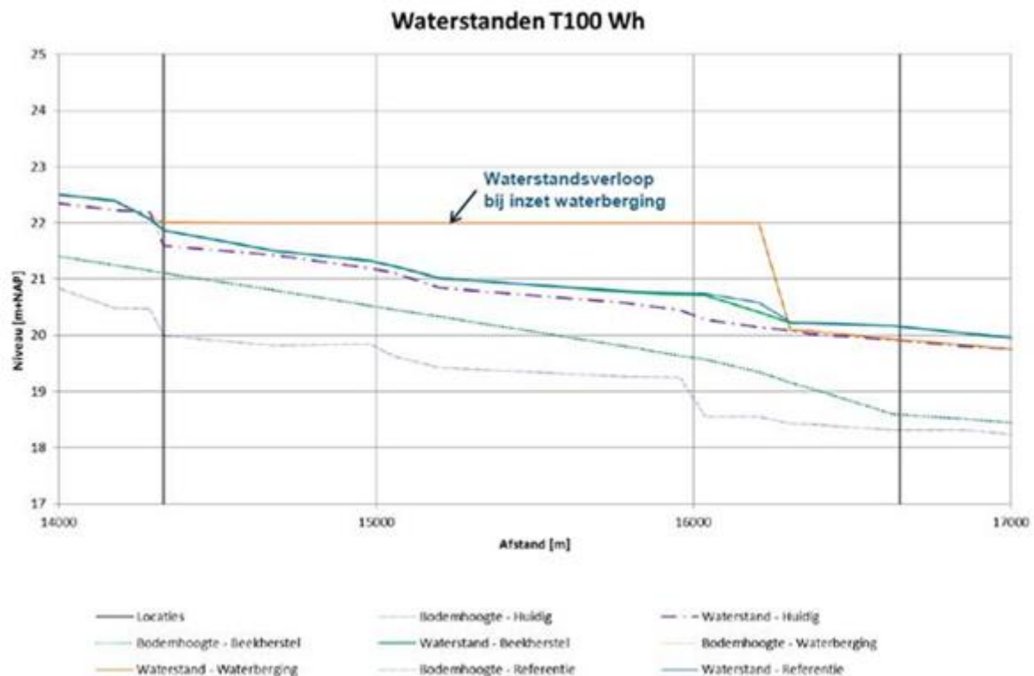
Figuur 3: Waterstanden T100 Wh
