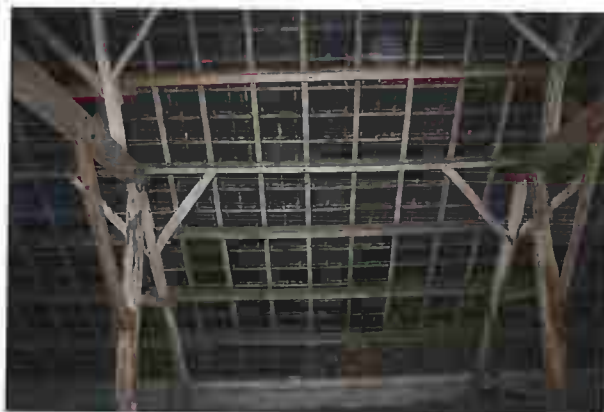
Oorspronkelijke en extra gordingen (pannenzijde)
