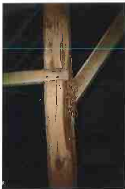
Detail: gespijkerde koppelbalk
