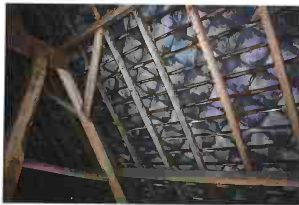
De oorspronkelijke gordingen (leienzijde)
