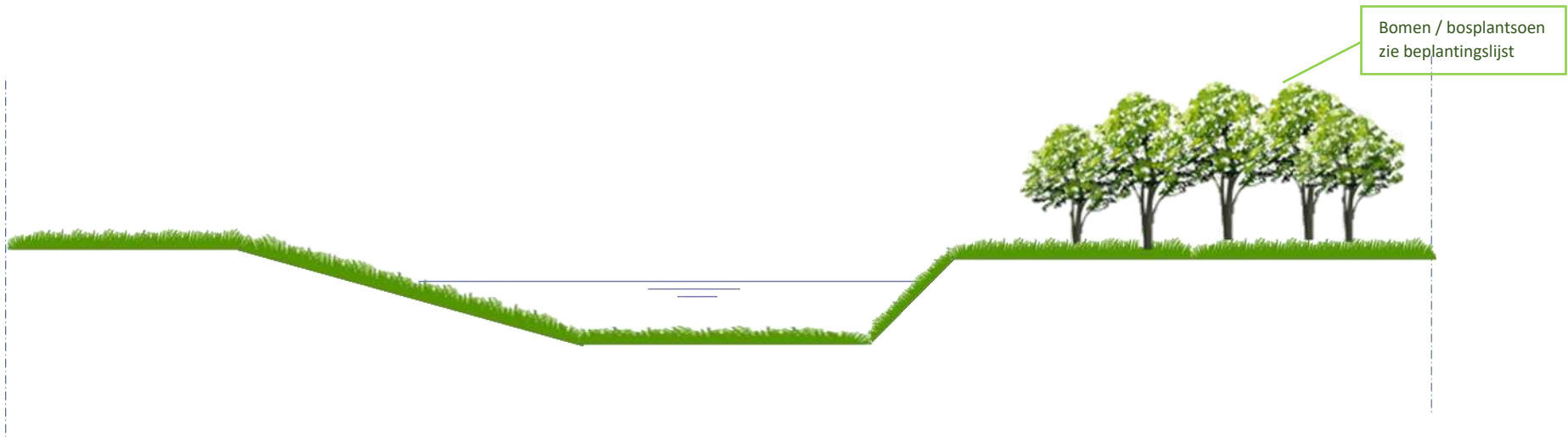
Doorsnede C-C
