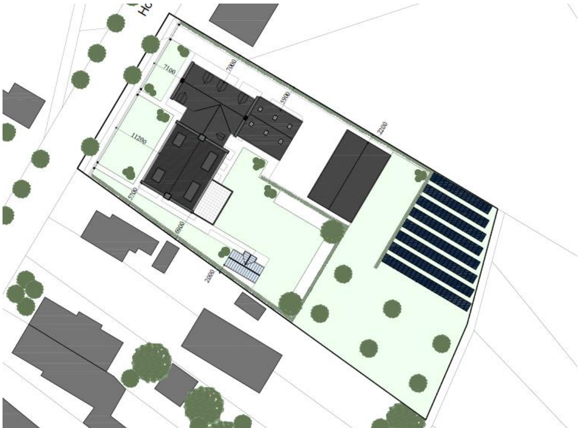
Figuur 3 Inrichtingstekening plangebied
