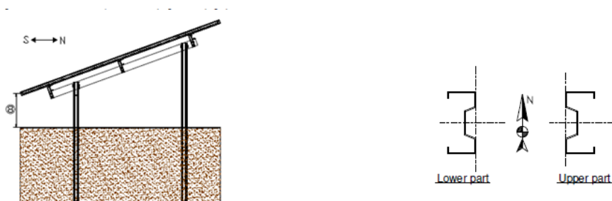
Figuur 6. Impressie fundering zonnepanelen.
