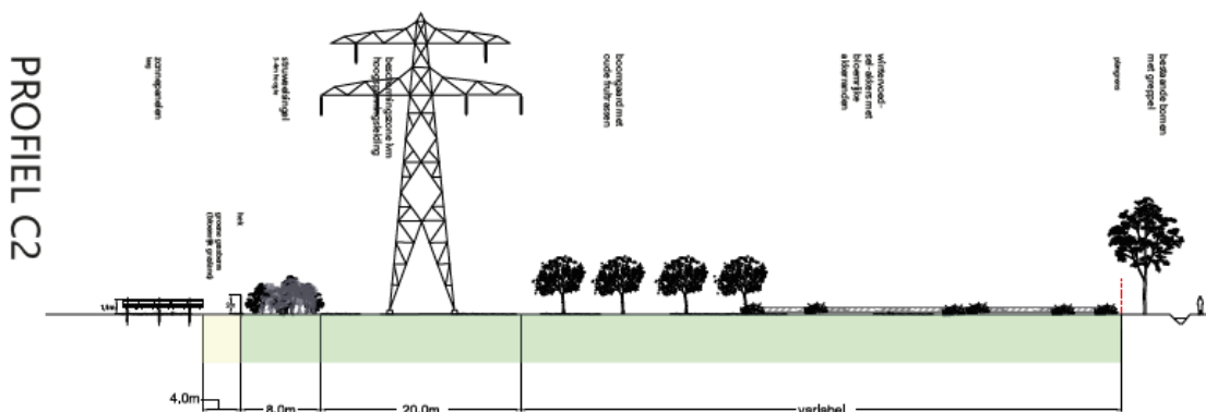
Figuur 8. Doorsnede 'C2' ter hoogte van de hoogspanningsleiding (bron: Haver Doeze).
