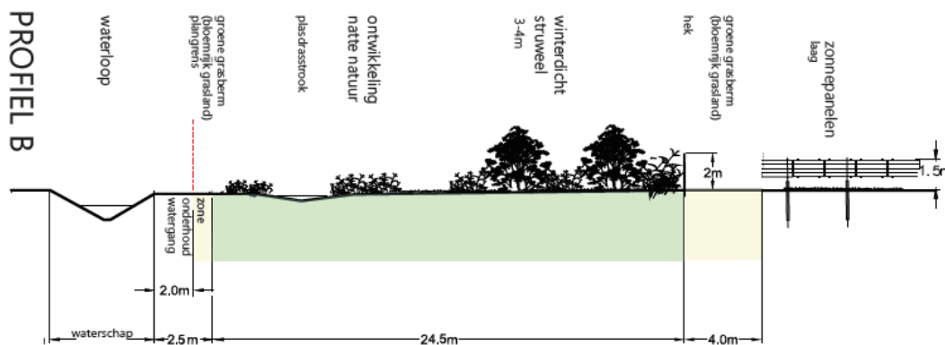
Figuur 9. Doorsnede 'B' aan de noordzijde van deelgebied 1 (bron: Haver Doeze).
