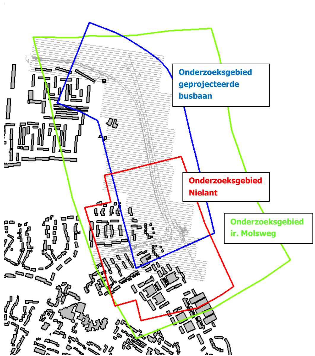
Figuur 1: Onderzoeksgebied Ir. Molsweg, Nielant en busbaan ten behoeve van het akoestisch onderzoek
