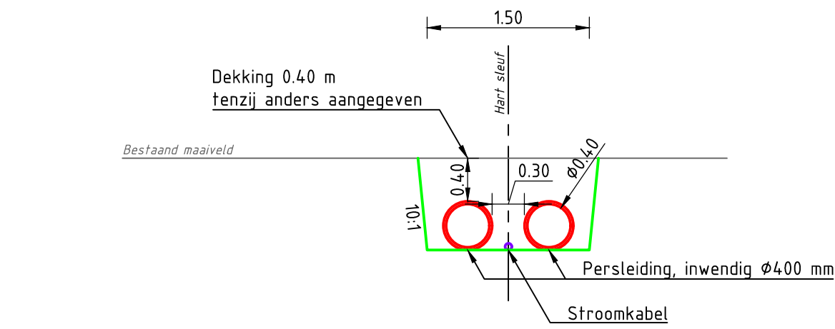
Principeprofiel sleuf SCHAAL 1 : 50
