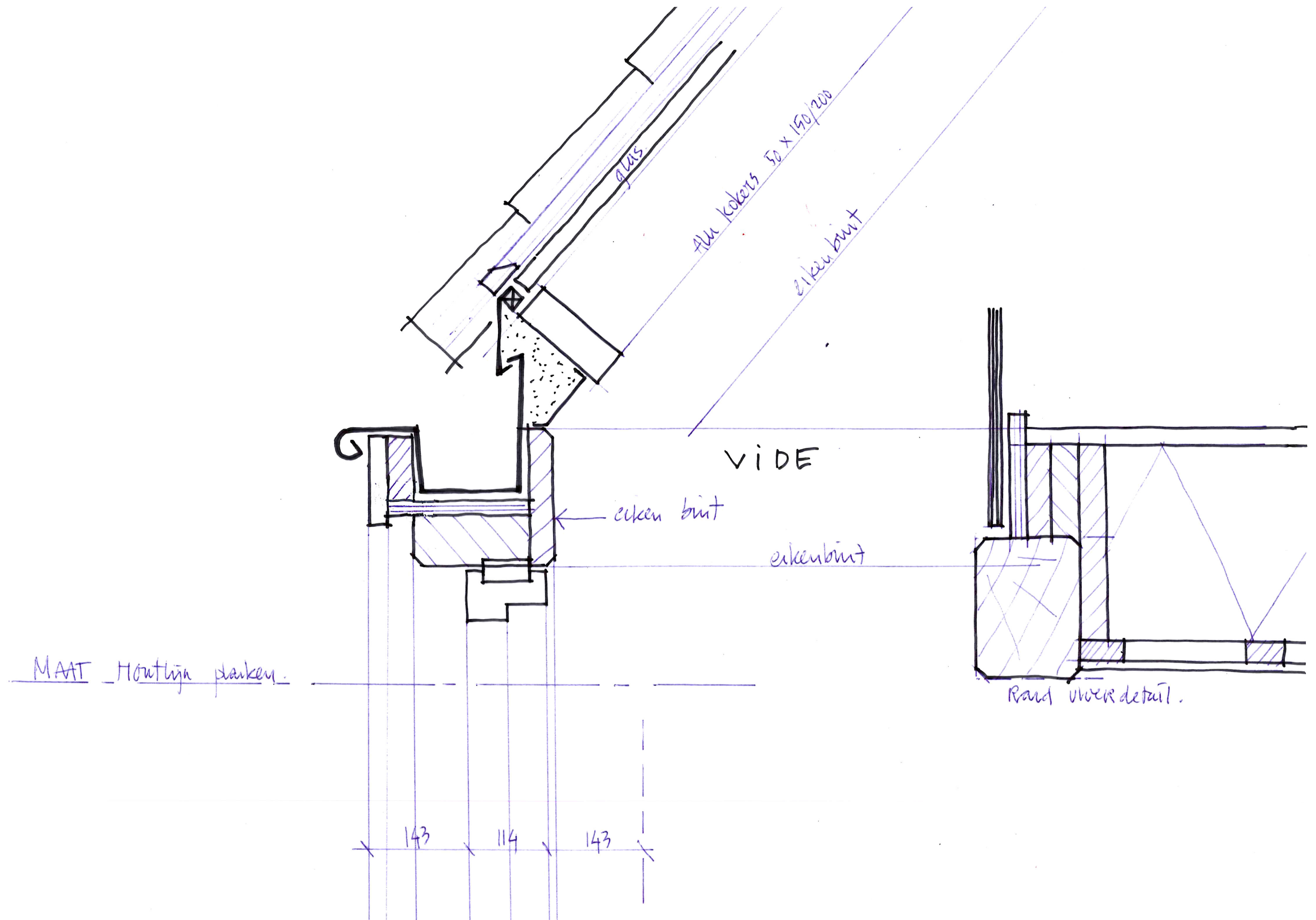
Detail 3 schaal 1:5
