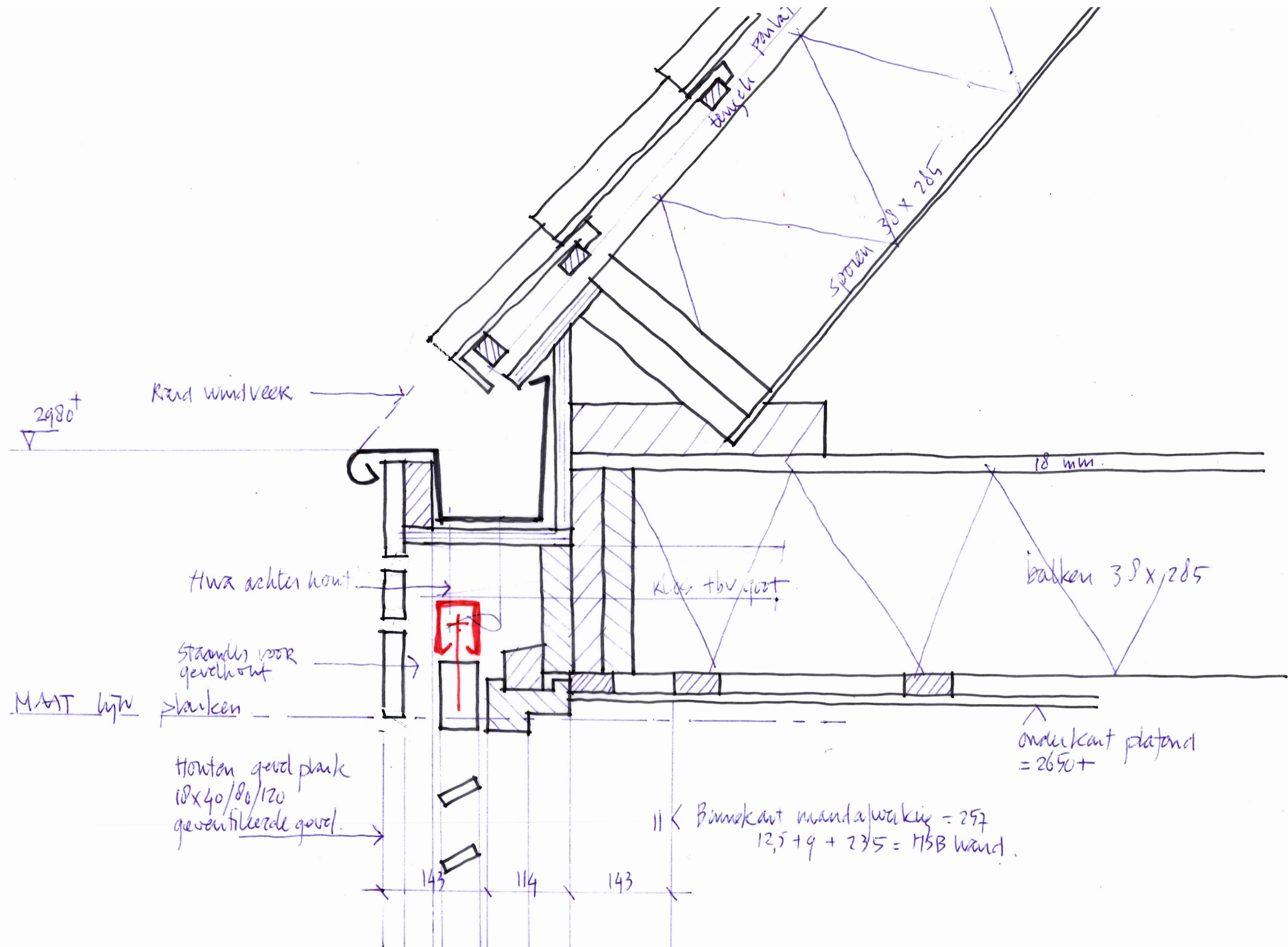
Detail 2 schaal 1:5
