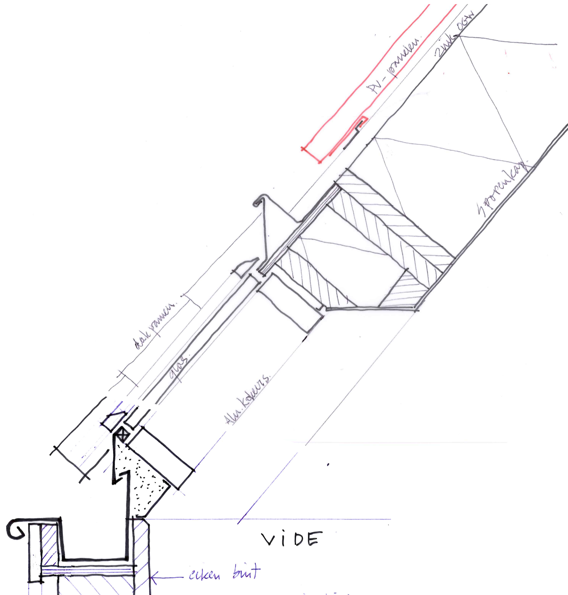
Detail 7 schaal 1:5
