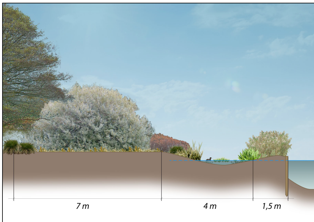
Figuur 5.2 Dwarsdoorsnede natuurvriendelijke oever en struweelrand (A-A')
