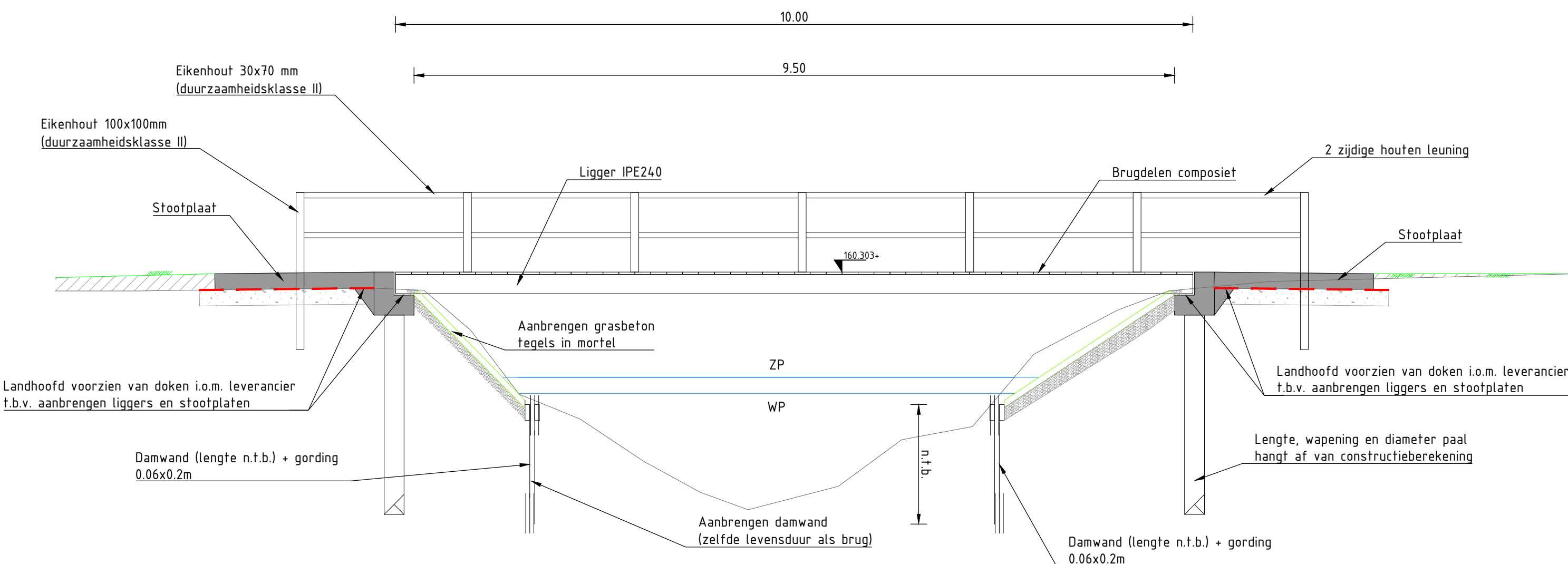
Principe profil 06 Voetgangersbrug schaal 1 : 50
