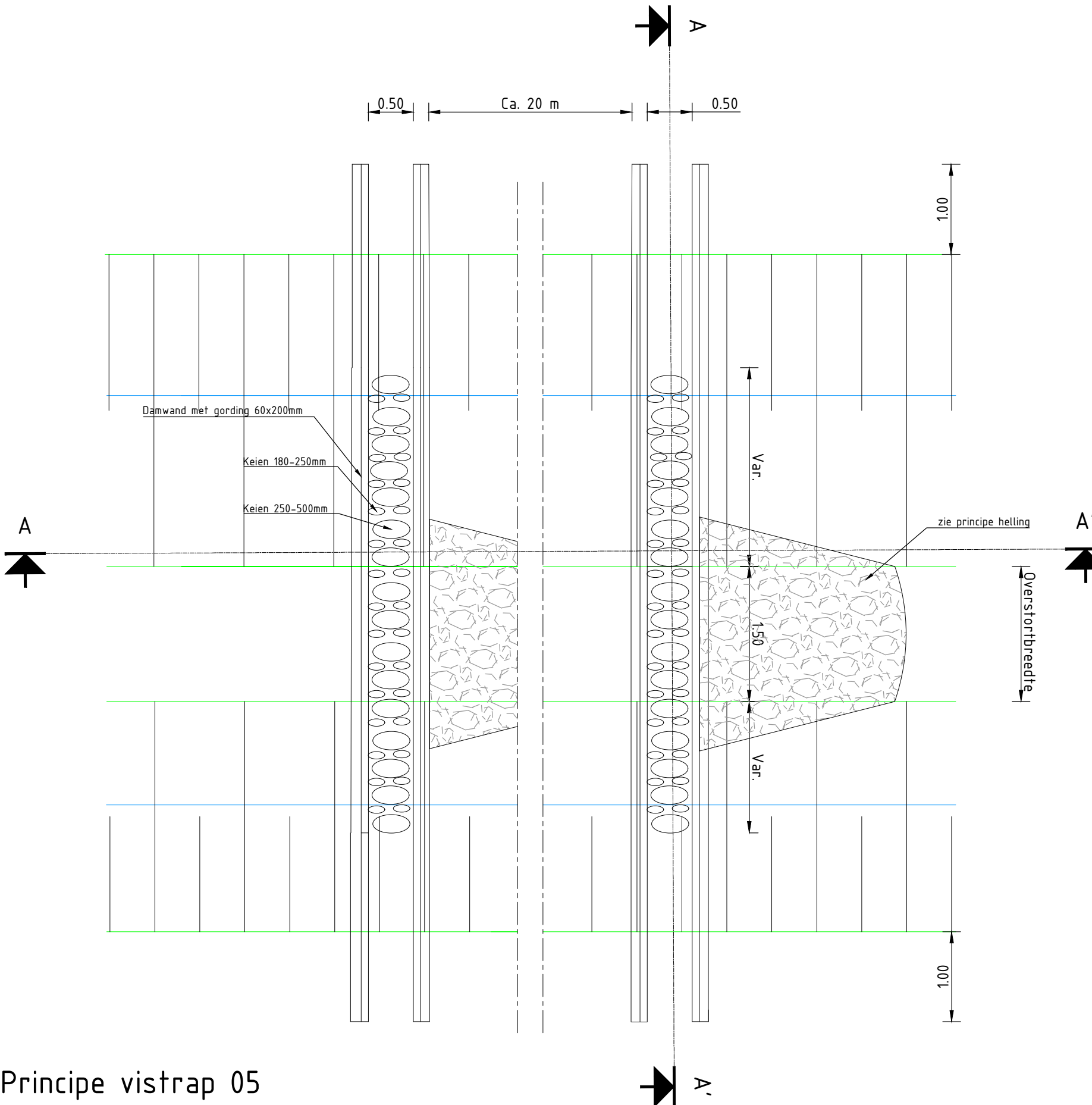
Principe vistrap 05 Boveenaanzicht schaal 1 : 50
