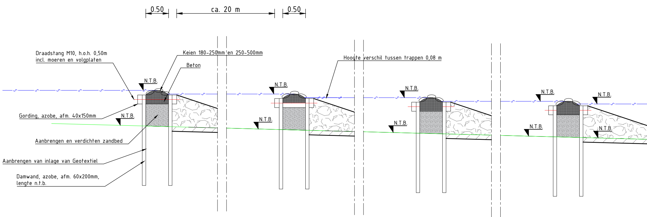
Principe lengteprofiel B - B' Vistrap, Aantal treden ## schaal 1 : 50
