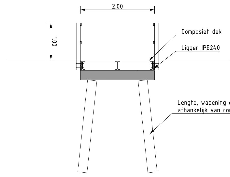
Dwarsprofiel A-A' Voetgangersbrug Schaal 150
