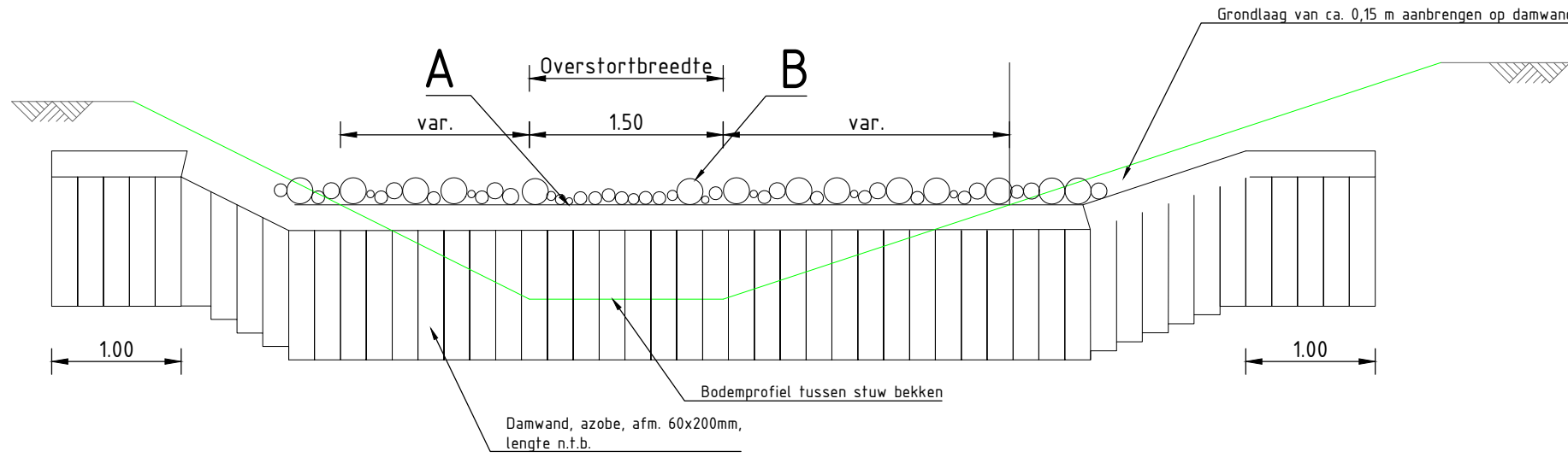
Principe dwarsprofiel A - A' Vistrap schaal 1 : 50
