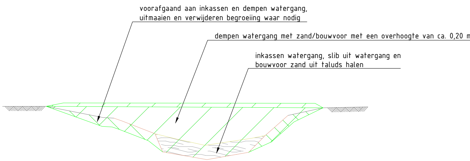
Principe profil 03 Te dempen watergang schaal 1 : 50
