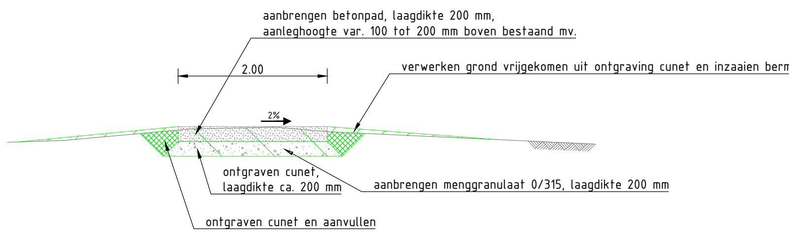
Principe profil Fietspad beton (look voor onderhoudsvoertuigen, dan met grasbetontegels) schaal 1 : 50
