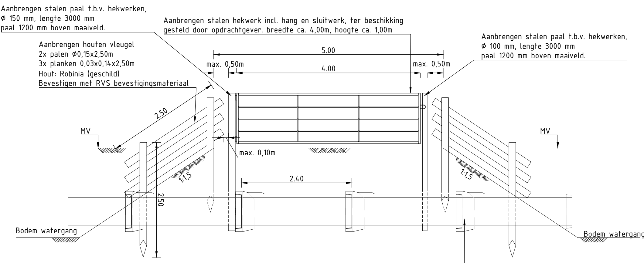
Principe profil Dan met duiker en hekwerk Schaal 150
